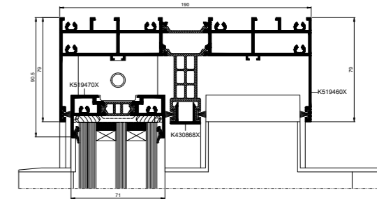
Oberer Schnitt der Tür
