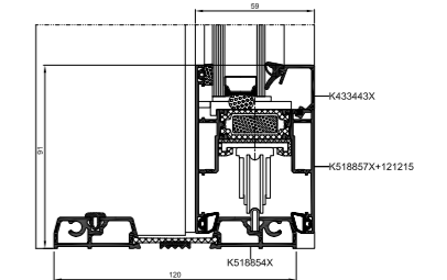
Schnitt durch Tür mit niedriger Schwelle
