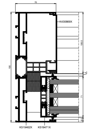
Seitlicher Schnitt der Tür
