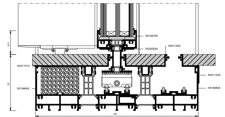
Schnitt Türunterseite
