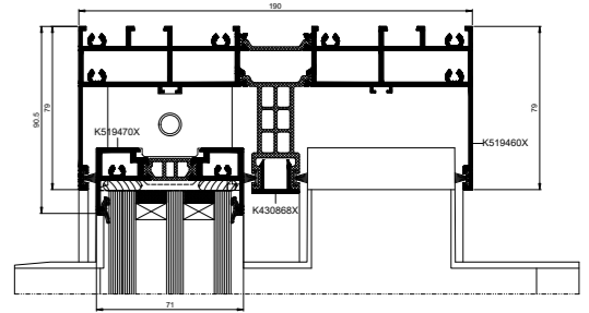
Schnitt Türoberseite
