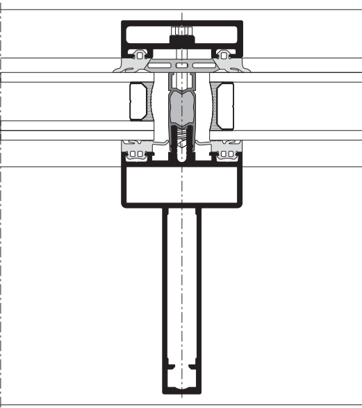
heroal C 50 ID Pfostenschnittdarstellung mit verschraubter Druckleiste (Stahlkontur)
