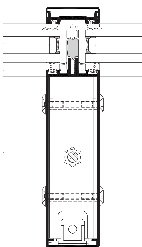
heroal C 50 PS Schnittdarstellung des Riegelspannsystems
