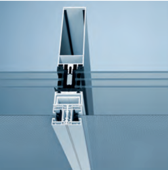
Fassaden teilintegriertes Sonnenschutzsystem heroal VS Z CS
