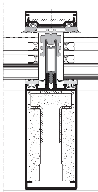
heroal C 50 FP Pfostenschnittdarstellung Brandschutzbereich
