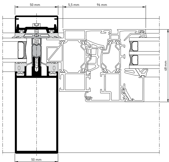
heroal C 50, řez sloupkem s osazovacím prvkem
