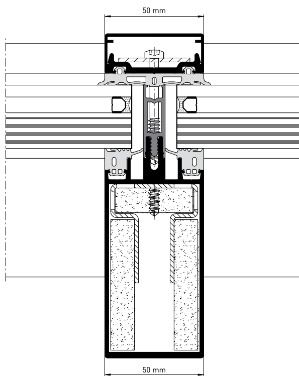
heroal C 50 FP, řez sloupkem v přechodové protipožární oblasti
