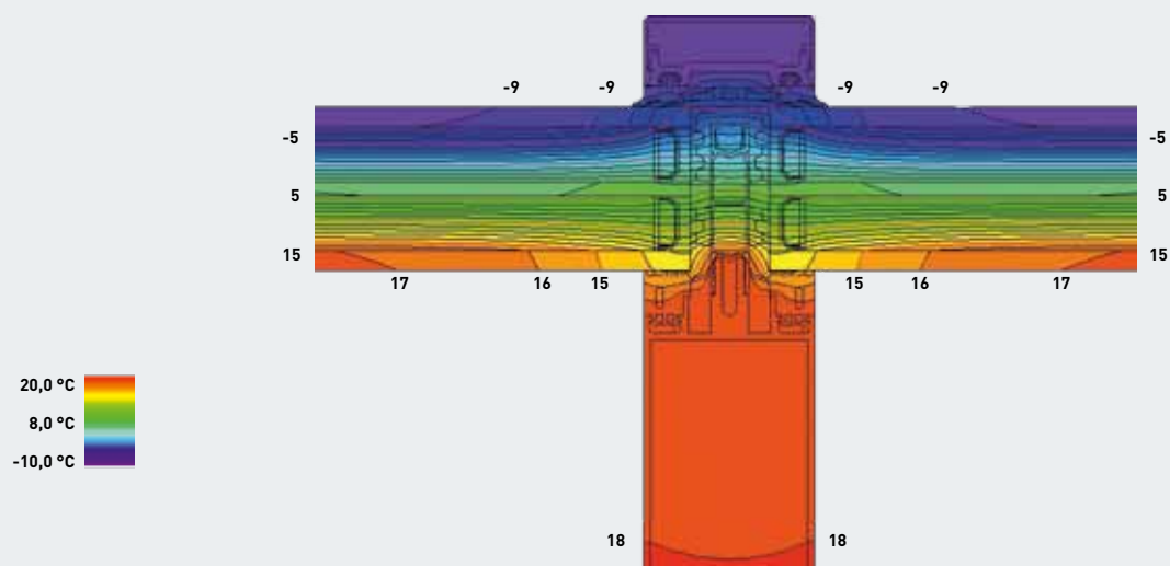
Průběh izoterm podle U_f EN ISO 10077-2
