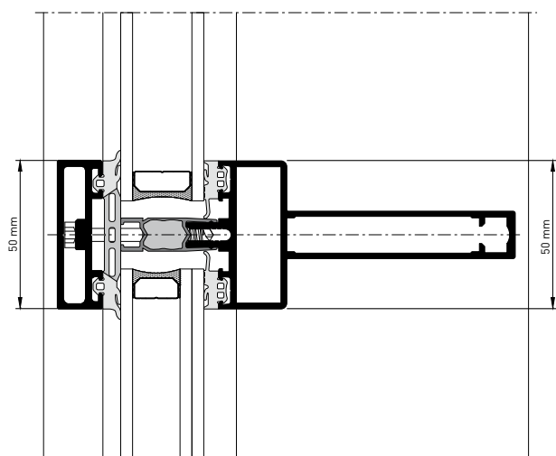
heroal C 50 ID, řez sloupkem s našroubovanou přitlačnou lištou (ocelová kontura)
