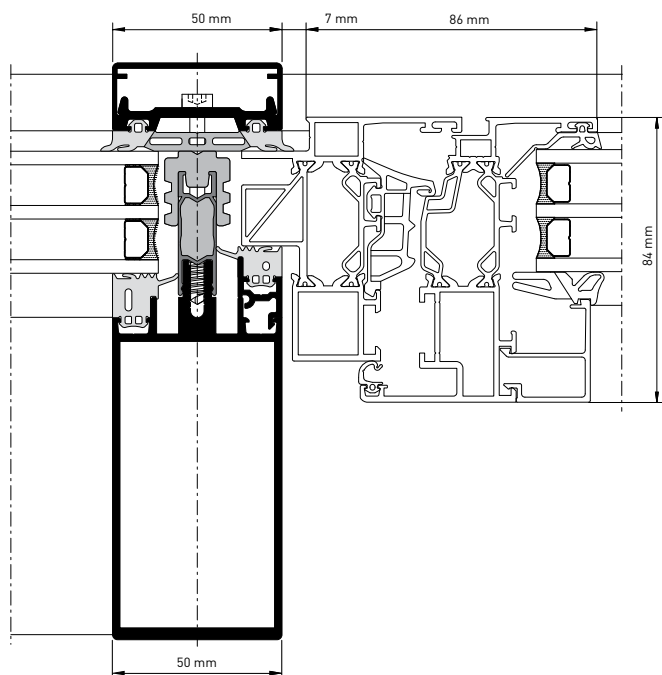
heroal C 50 HI, řez sloupkem s osazovacím prvkem
