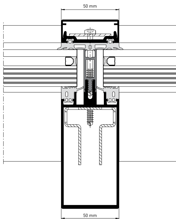
heroal C 50 FP, řez sloupkem v protipožární oblasti
